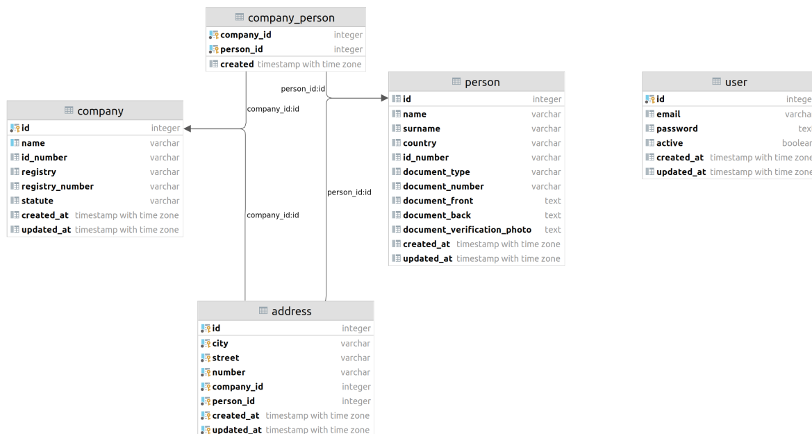
Obr. 4.3: Ukážka dátového modelu
