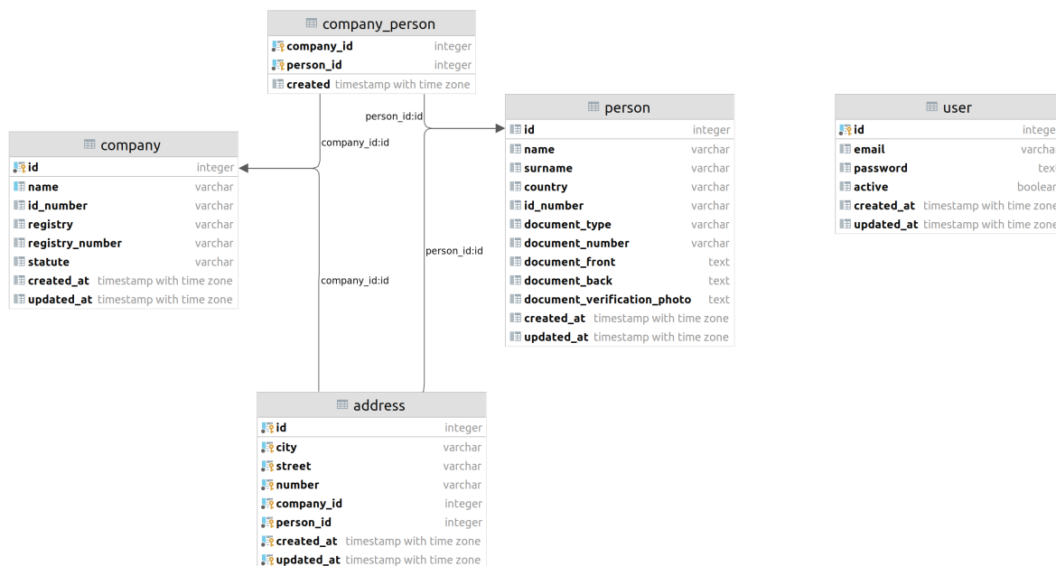
Obr. 3.2: Dátový model backendu
