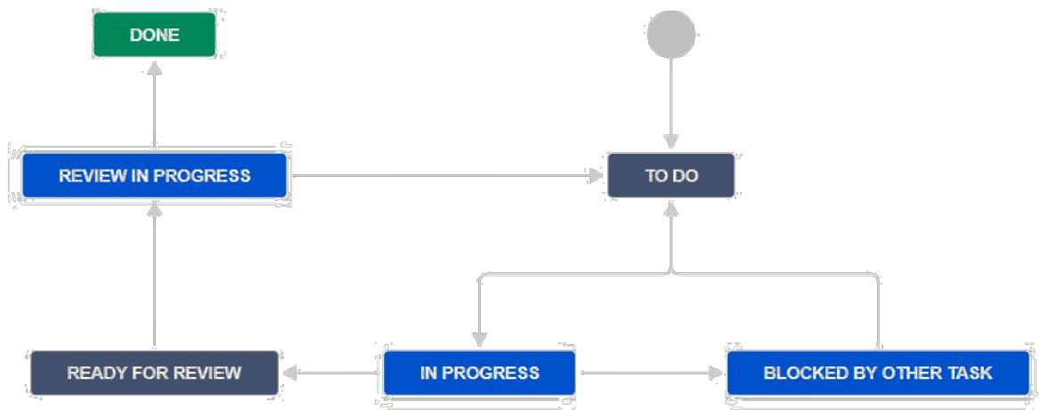
Obrázok 1. - Azure Workflow
