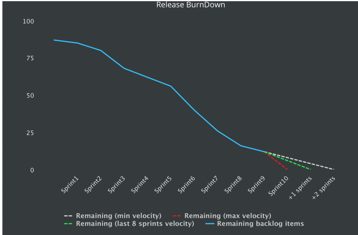
Obrázok 30: Burndown chart
