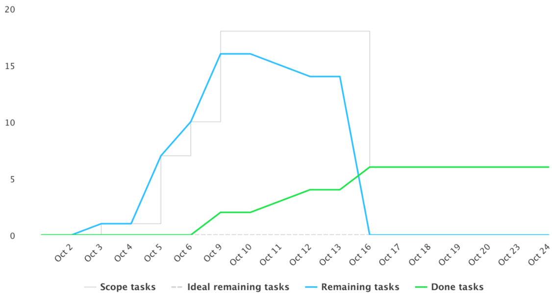
Obrázok 3: Burndown Chart
