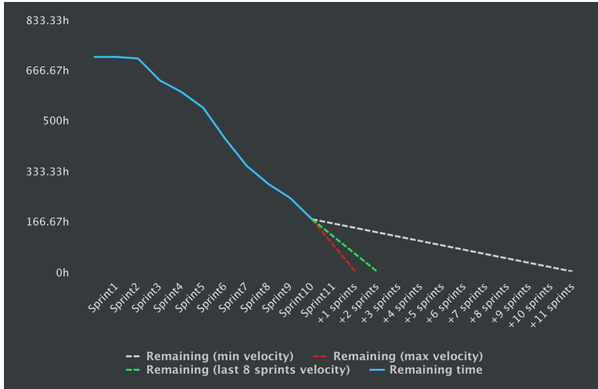
Obrázok 45: Burndown chart
