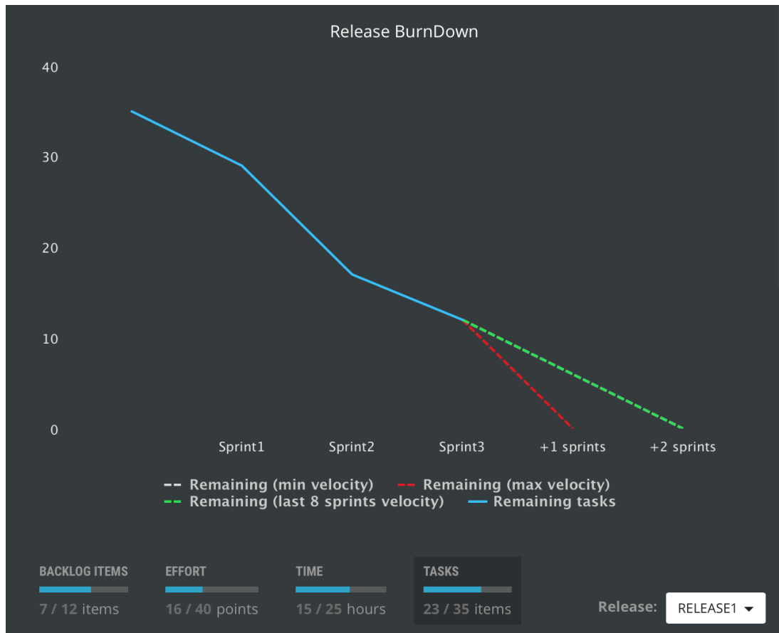
Obrázok 10: Release Burndown
