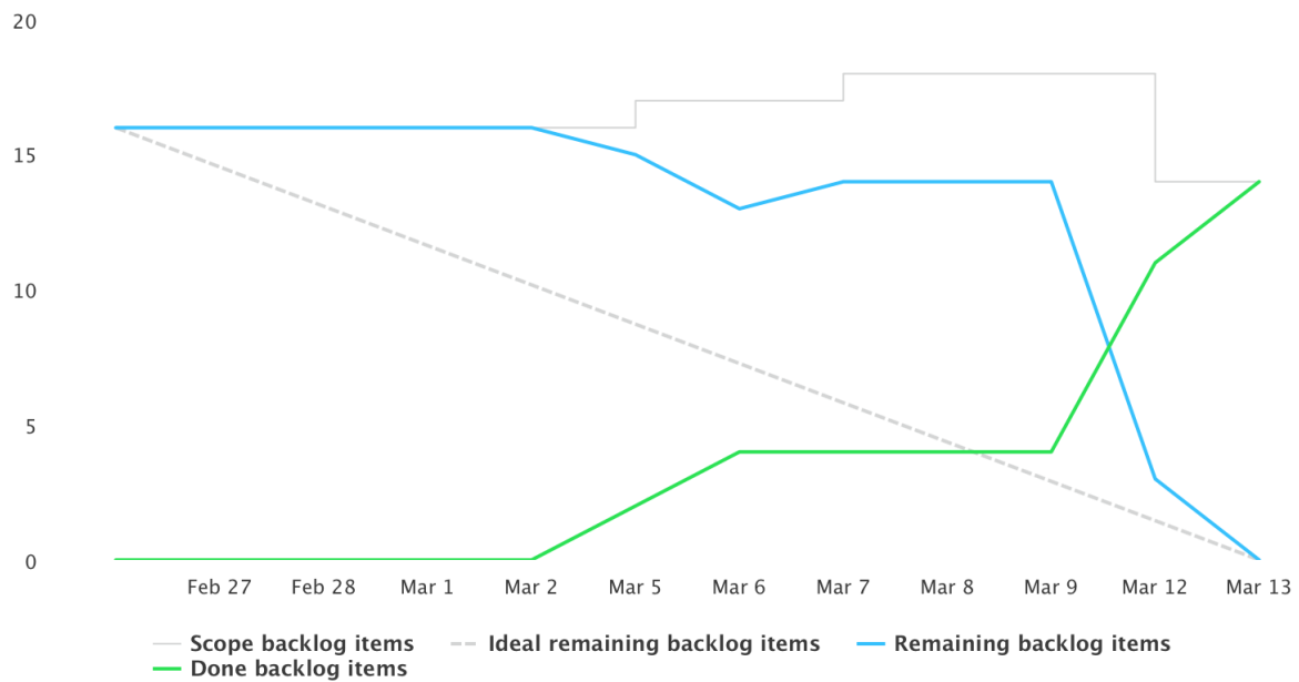
Obrázok 33: Burndown chart
