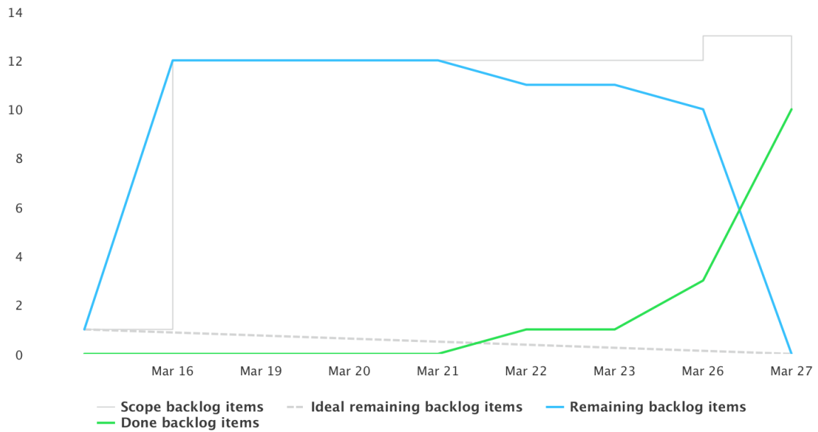
Obrázok 38: Burndown chart
