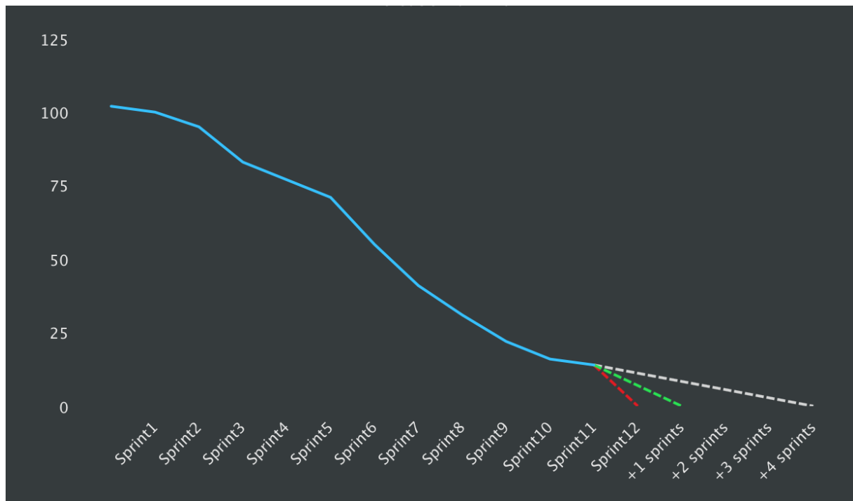
Obrázok 50: Burndown chart
