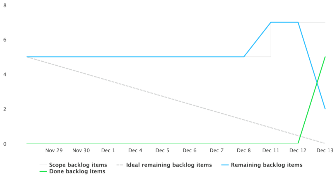
Obrázok 23: Burndown chart
