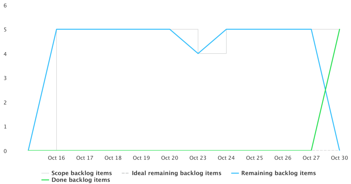
Obrázok 8: Burndown Chart
