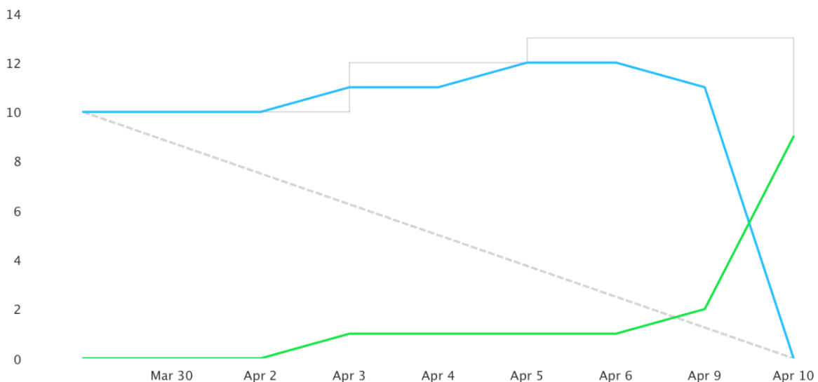
Obrázok 48: Burndown chart
