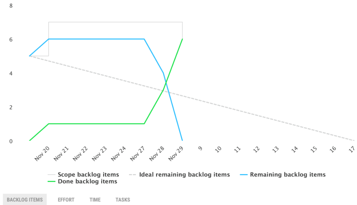
Obrázok 18: Burndown chart
