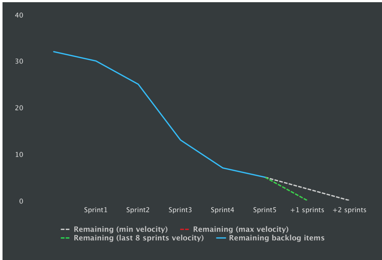
Obrázok 20: Burndown chart
