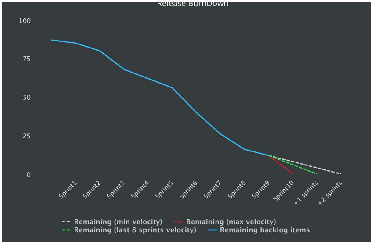
Obrázok 35: Burndown chart
