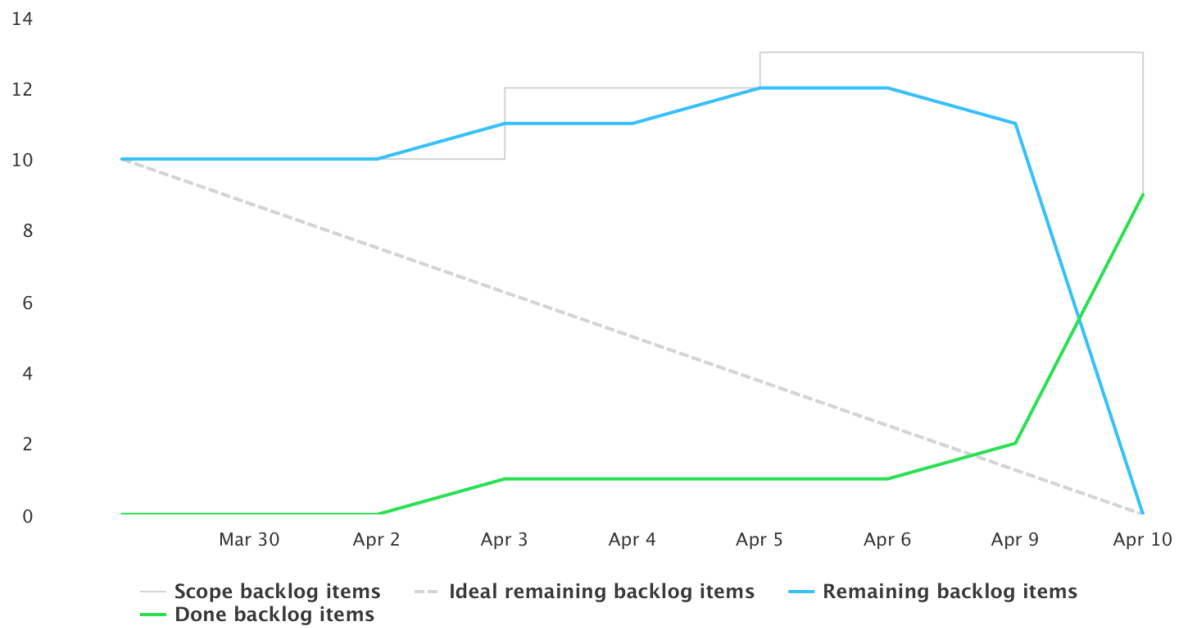
Obrázok 43: Burndown chart
