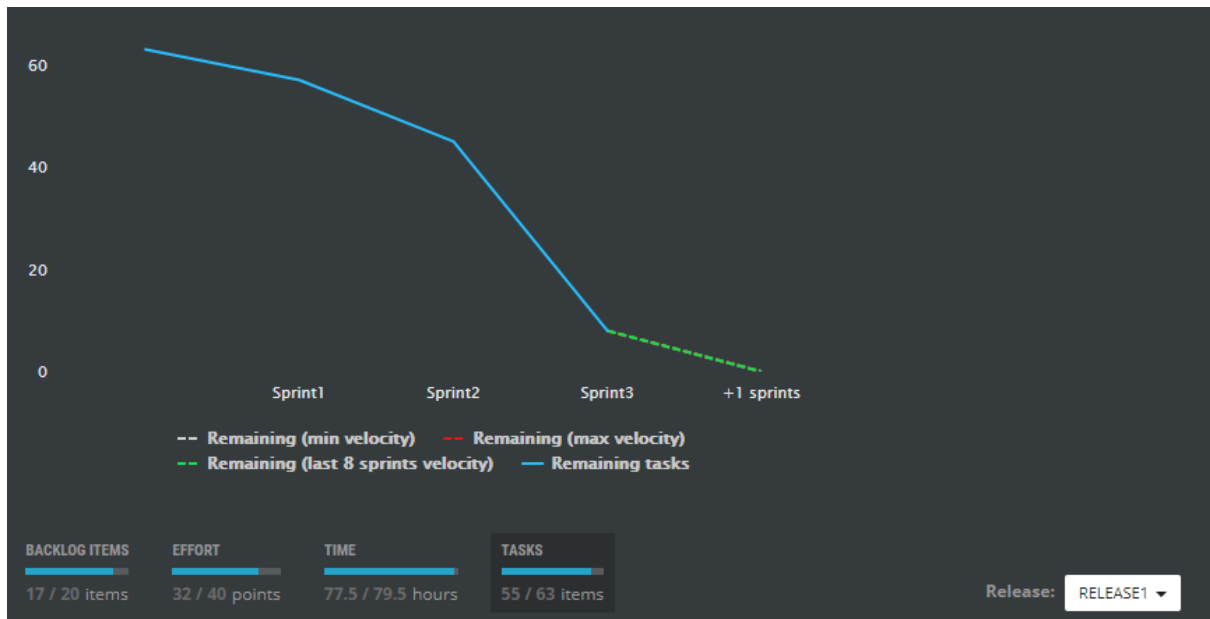
Obrázok 15: Burndown chart
