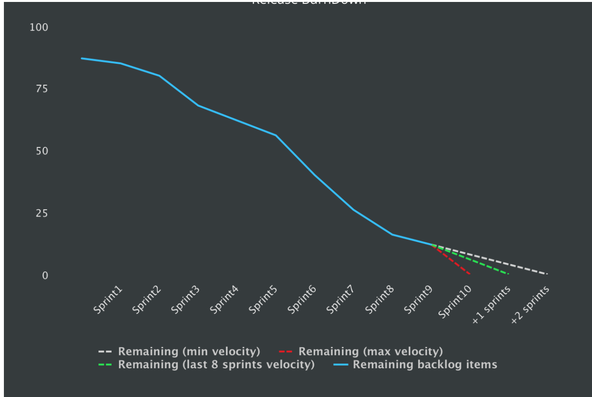
Obrázok 40: Burndown chart
