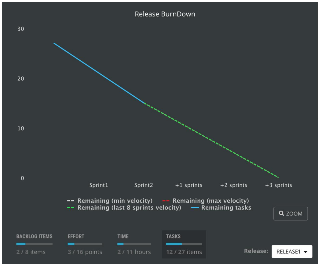
Obrázok 5: Release Burndown
