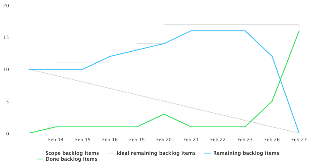
Obrázok 28: Burndown chart
