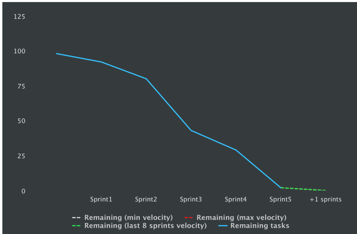
Obrázok 25: Burndown chart
