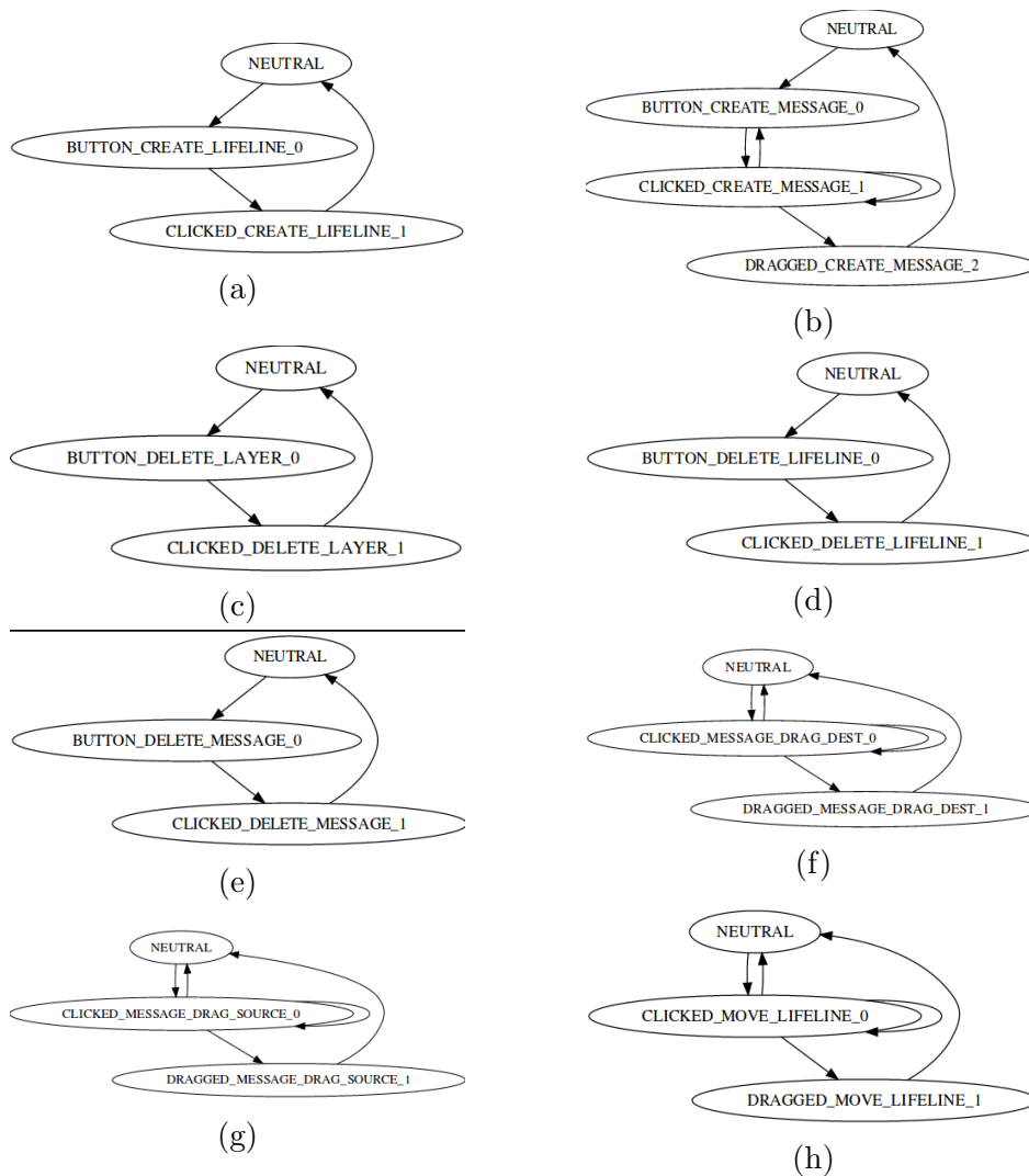
Obr. 5: Stavové diagramy aplikácie: (a) vytvorenie lifelinu, (b) vytvorenie správy, (c) vymazanie vrstvy, (d) vymazanie lifelinu, (e) vymazanie správy, (f) posunutie konca správy, (g) posunutie začiatku správy, (h) posunutie lifelinu
