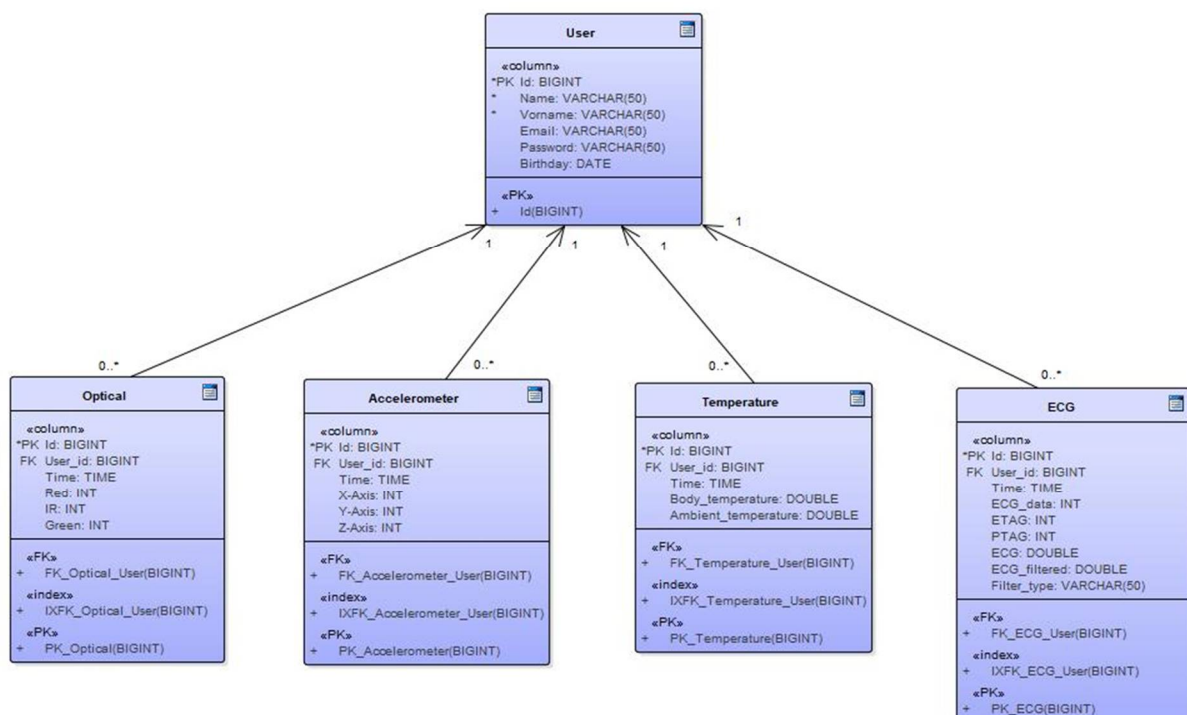
Obrázok 2: Dátový model
