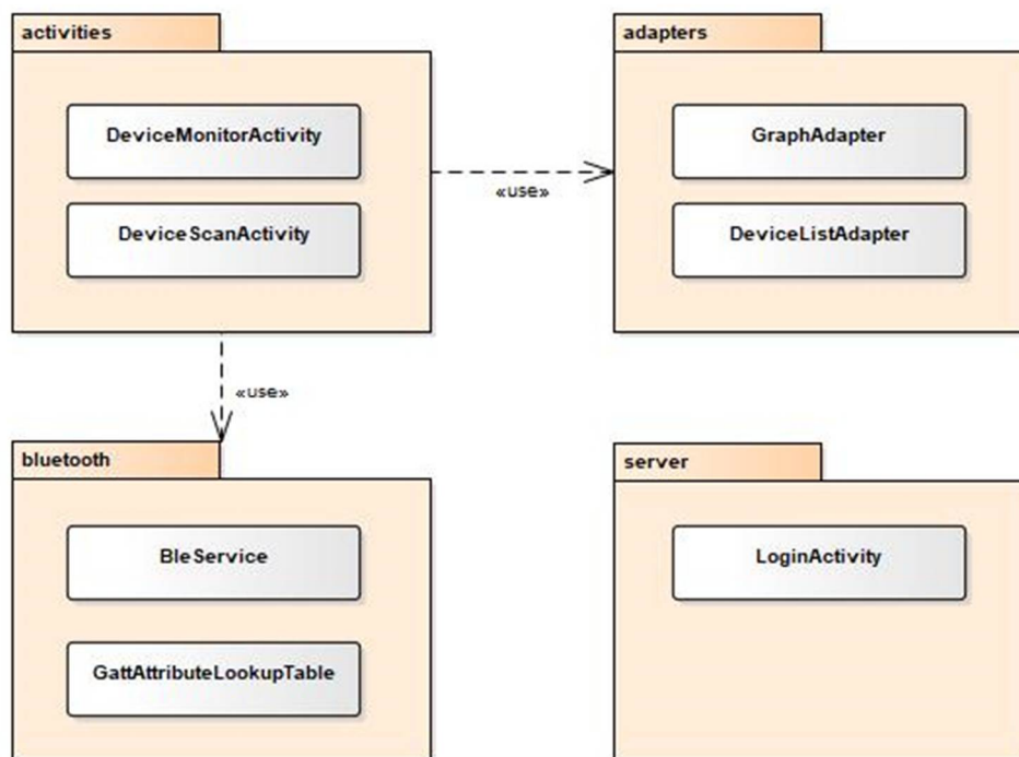
Obrázok 5: Diagram balíkov
