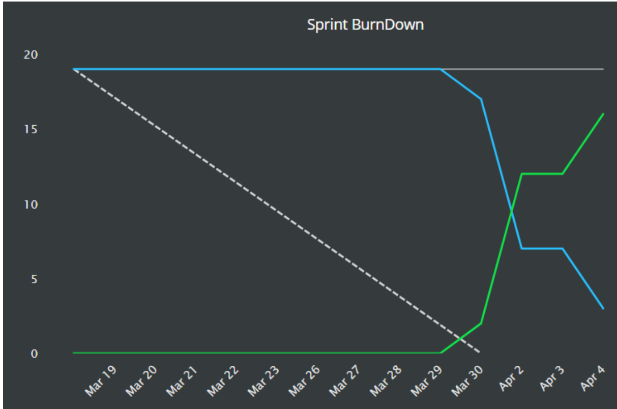
Obrázok 1 BurnDown graf z ôsmeho šprintu
