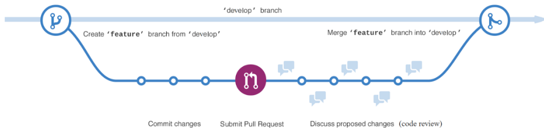
Obrázok 11: Práca na novej funkcionalite z pohľadu verziovacieho systému podľa Git metodiky
