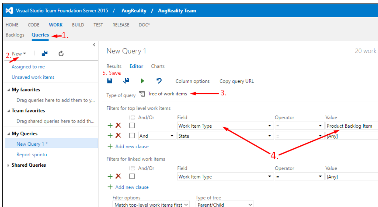
Obrázok 13: Vytváranie query za účelom exportu úloh zo systému TFS
