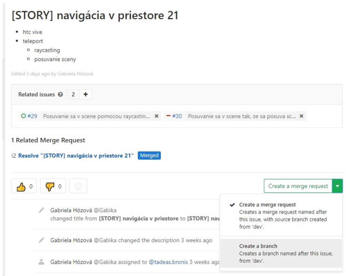
Obrázok č. 2: Vytvorenie vetvy
