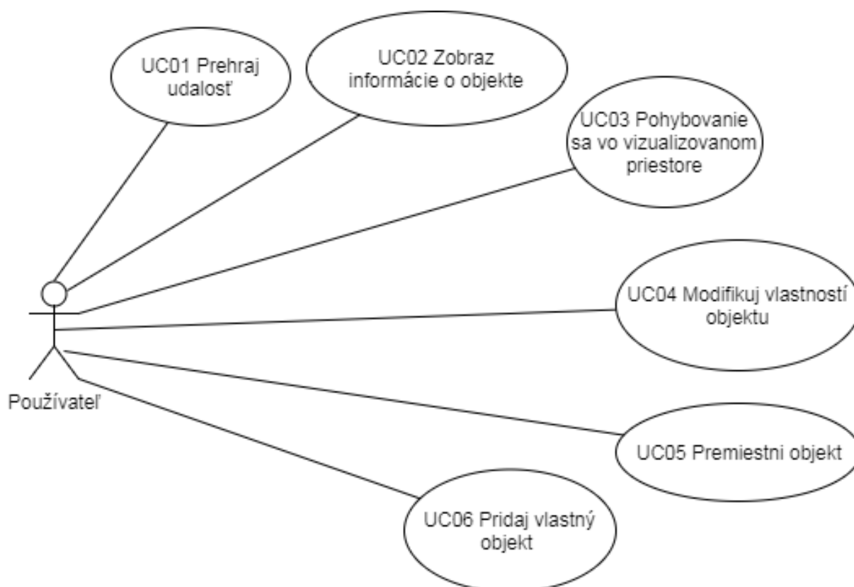
Obrázok č. 8: Diagram prípadov použitia
