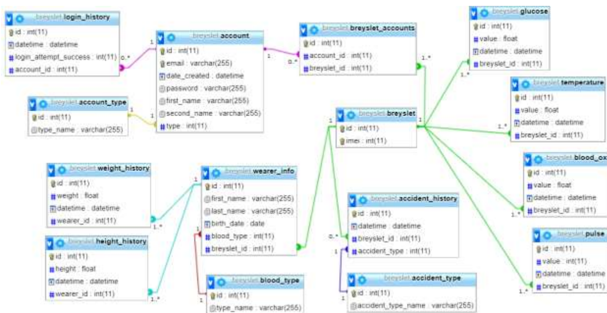
Obr. 4 - Fyzický dátový model
