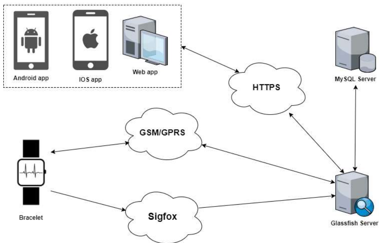
Obr. 3 - Architektúra systému
