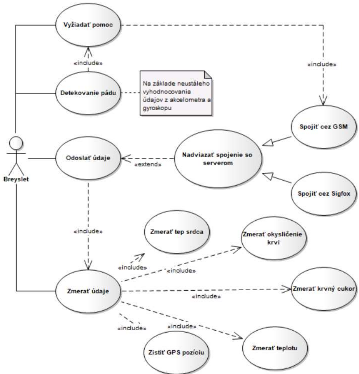
Obr. 1 - Diagram prípadov použitia - náramok Breyset
