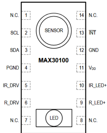
Obr. 6 - rozloženie pinov modulu MAX30100
