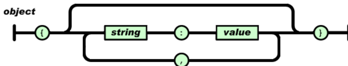
Obr. 7 - Štruktúra objektu vo formáte JSON 5
