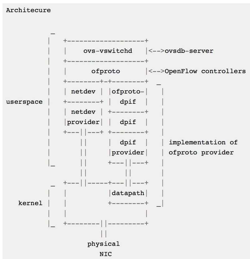
Obr. 4. Architektúra OVS
