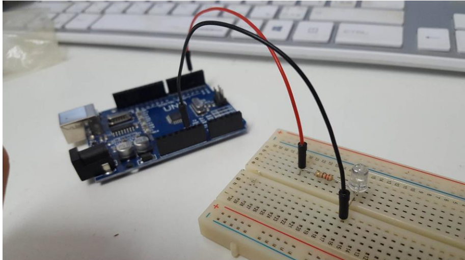
Obrázok 1 Testovacie zapojenie
