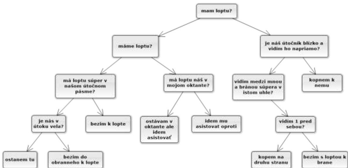
Obrázok 5.13 rozhodovací strom obrancu v oktante 1L (napravo – true, naľavo - false)
