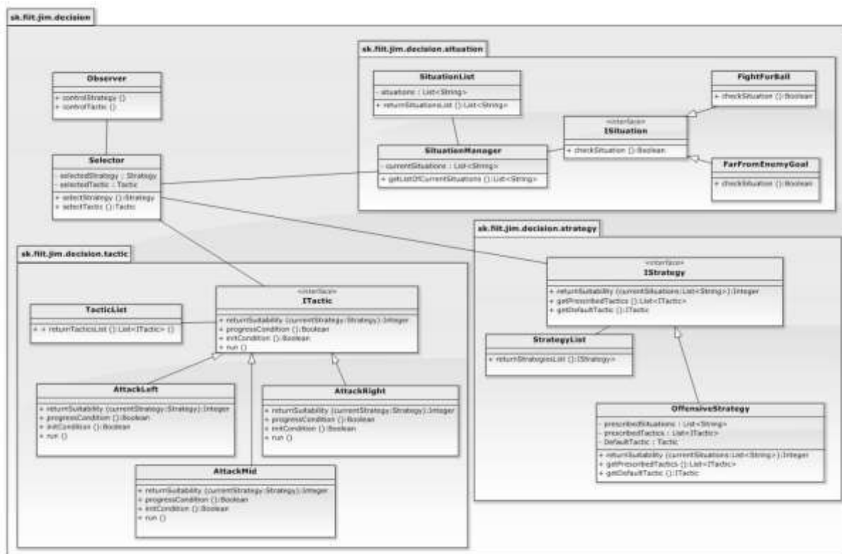
Obrázok A.2 Diagram tried súčasnej architektúry
