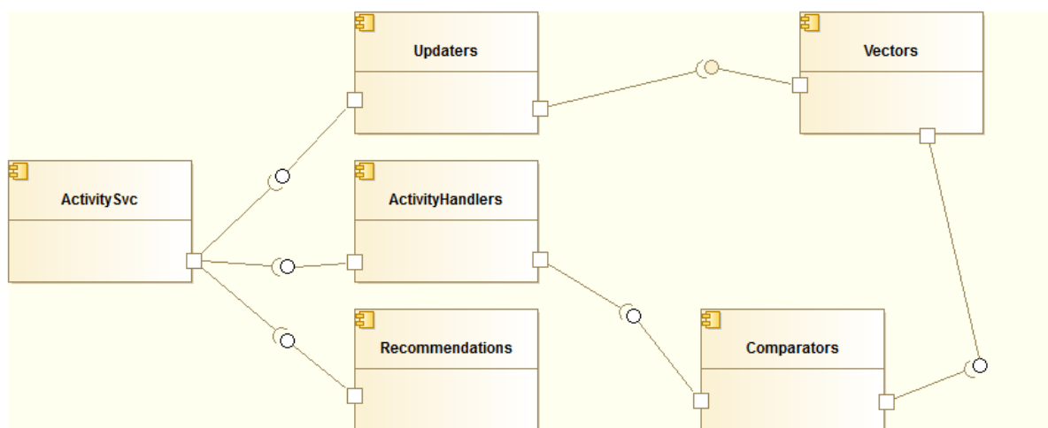
OBRÁZOK 33 - KOMPONENTY APLIKÁCIE
