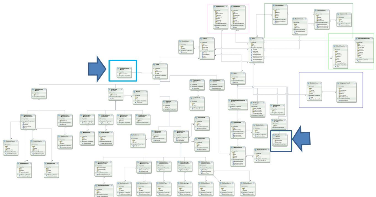
OBRÁZOK 45 DÁTOVÝ MODEL
