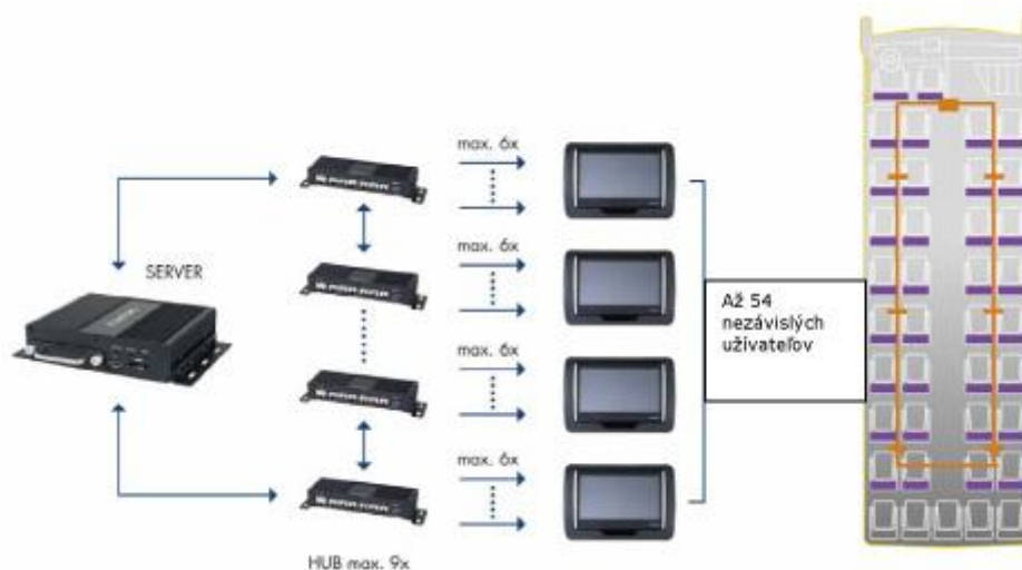
Obr. 2: Architektúra zapojenia digitálneho MOD systému
