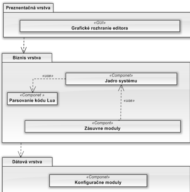
Obr. 3 Architektúra programu
