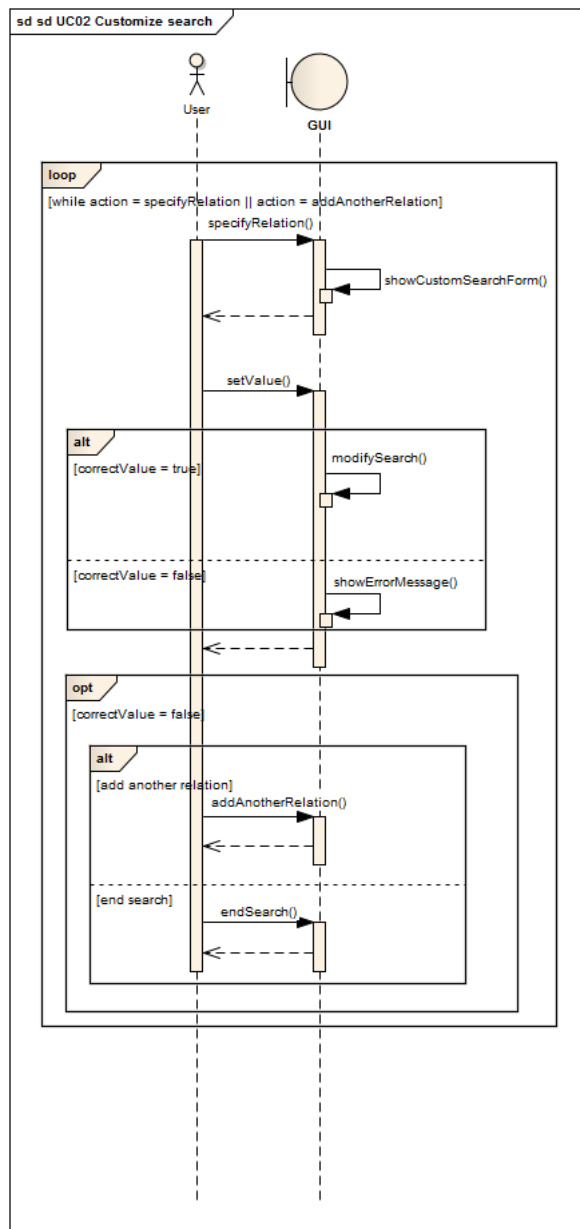
Obr. 4.3: Sekvenčný diagram pre UC02 Upravenie vyhľadávania
