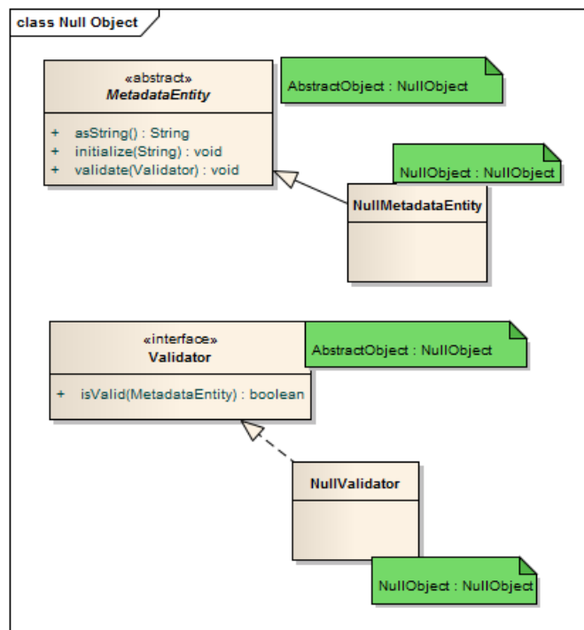
Obr. E.2: Null object
