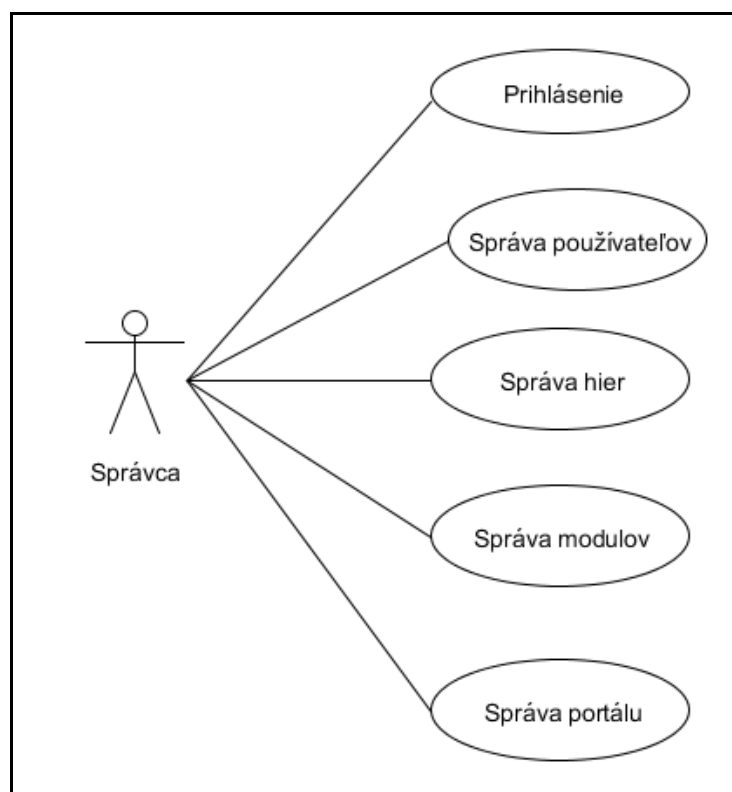
Obr. 4 Diagram prípadov použitia pre správca
