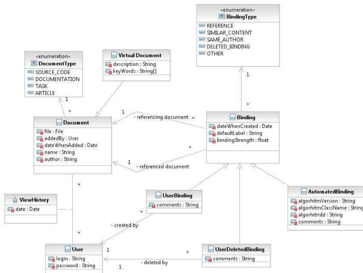
Obr. 10. Dátový model
