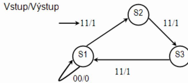
Obr. 1.15: Stavový automat
