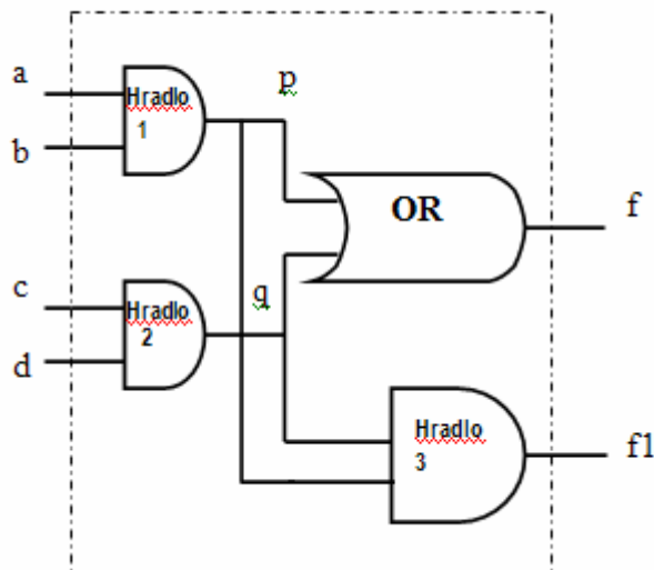
Obr. 1.14: Jednoduchý obvod
