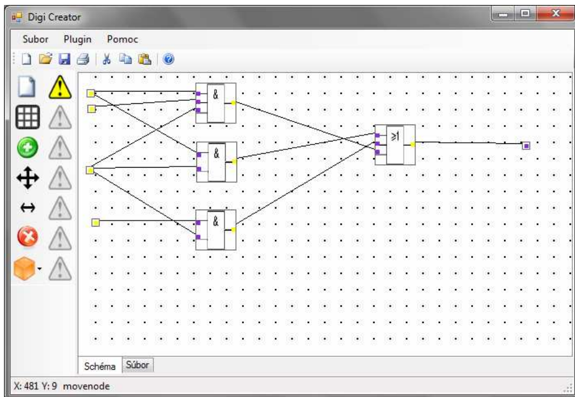
Obr.3: Grafický editor
