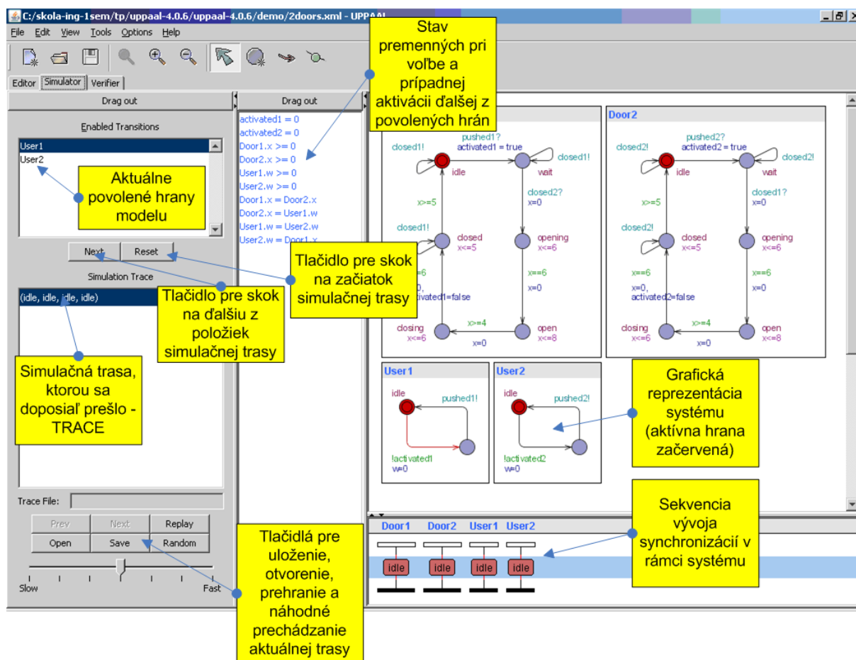
Obrázok 2 - Simulátor systému
