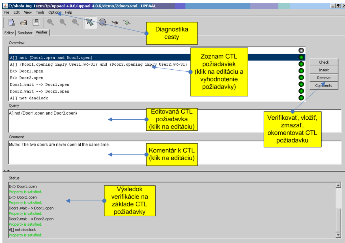
Obrázok 3 - Verifikátor systému
