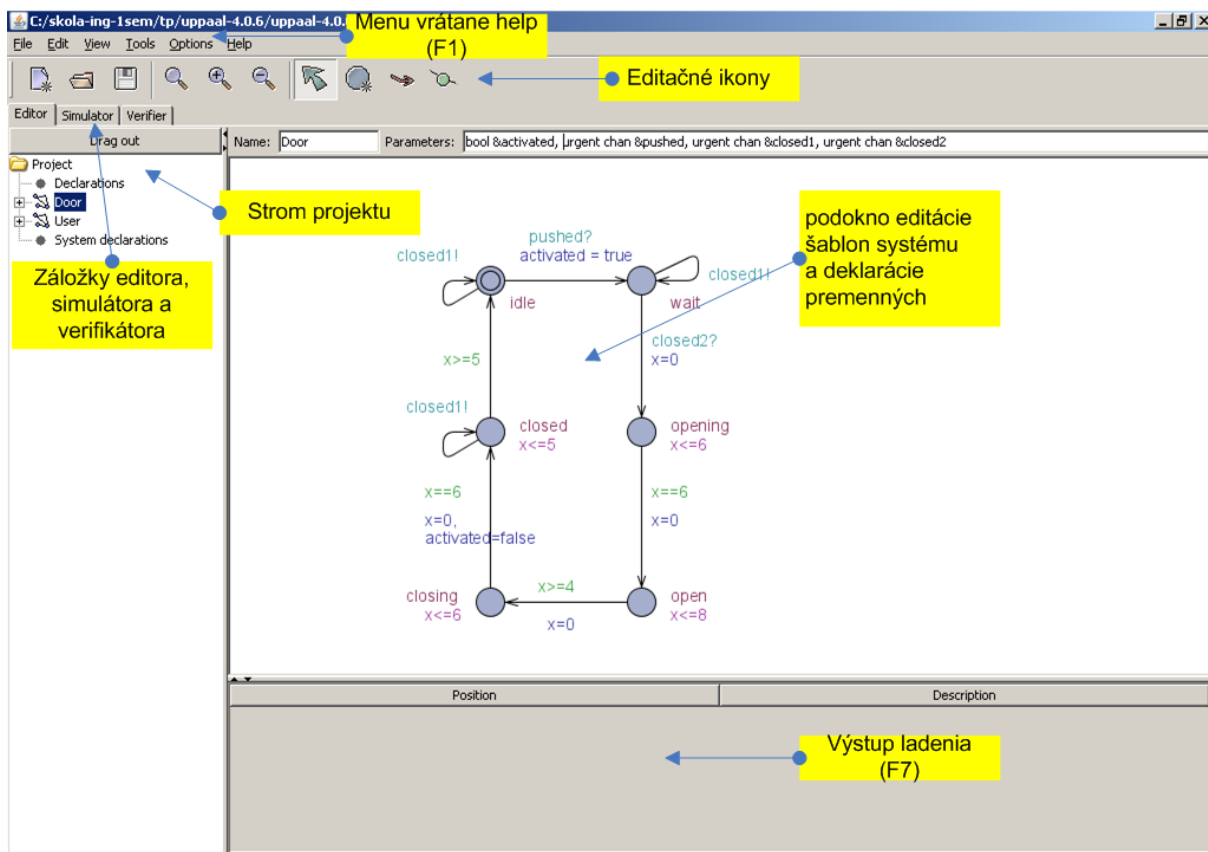
Obrázok 1- Editor systému
