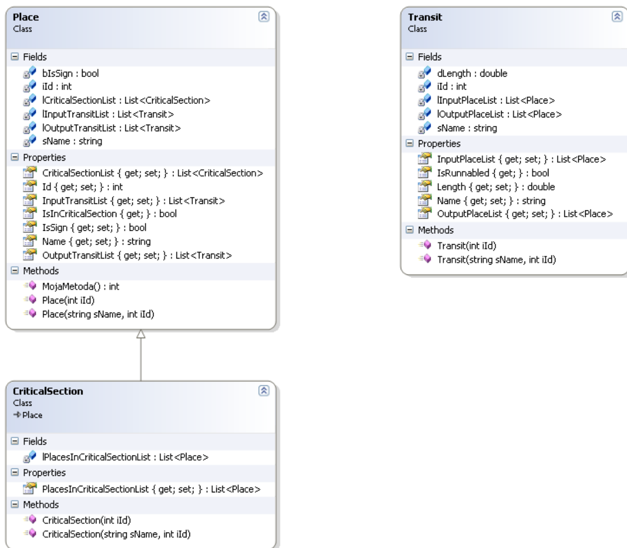
Dátový model
