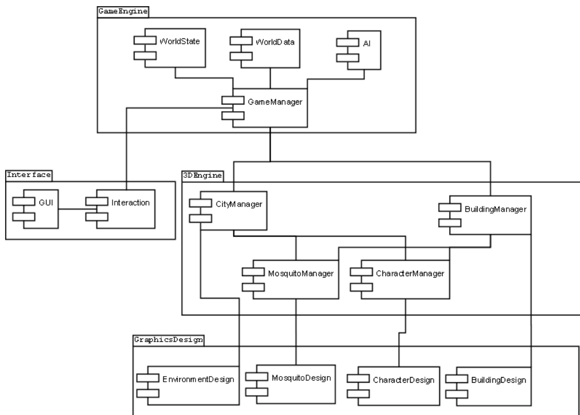
Obr. 8. Architektúra aplikácie.
