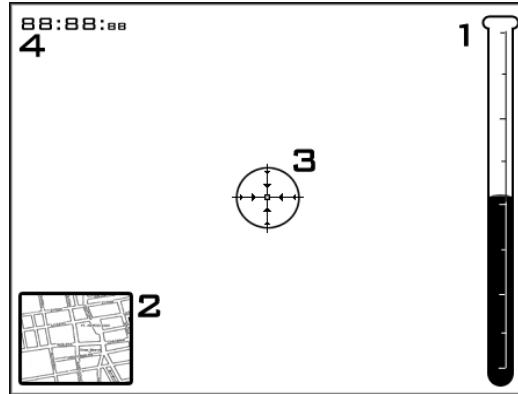
Obr. 12. Návrh GUI.
