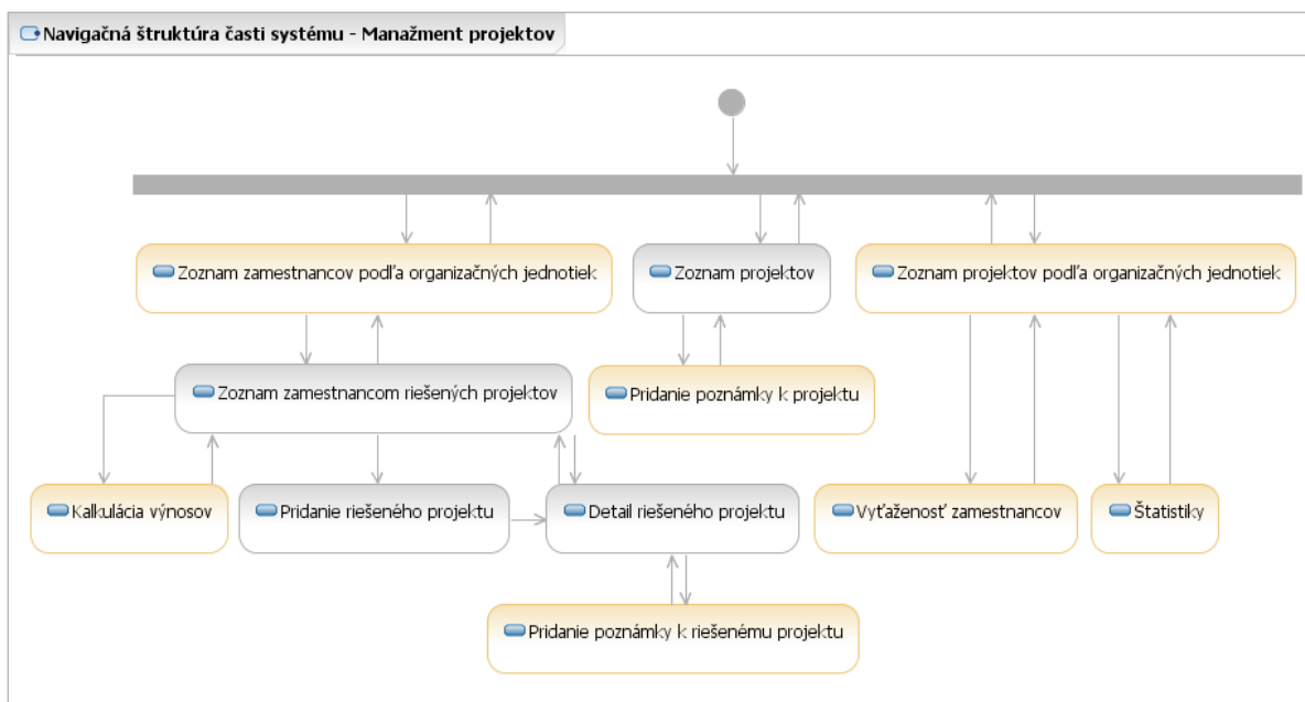
Obr. 28. Navigačná štruktúra časti Manažment projektov.
