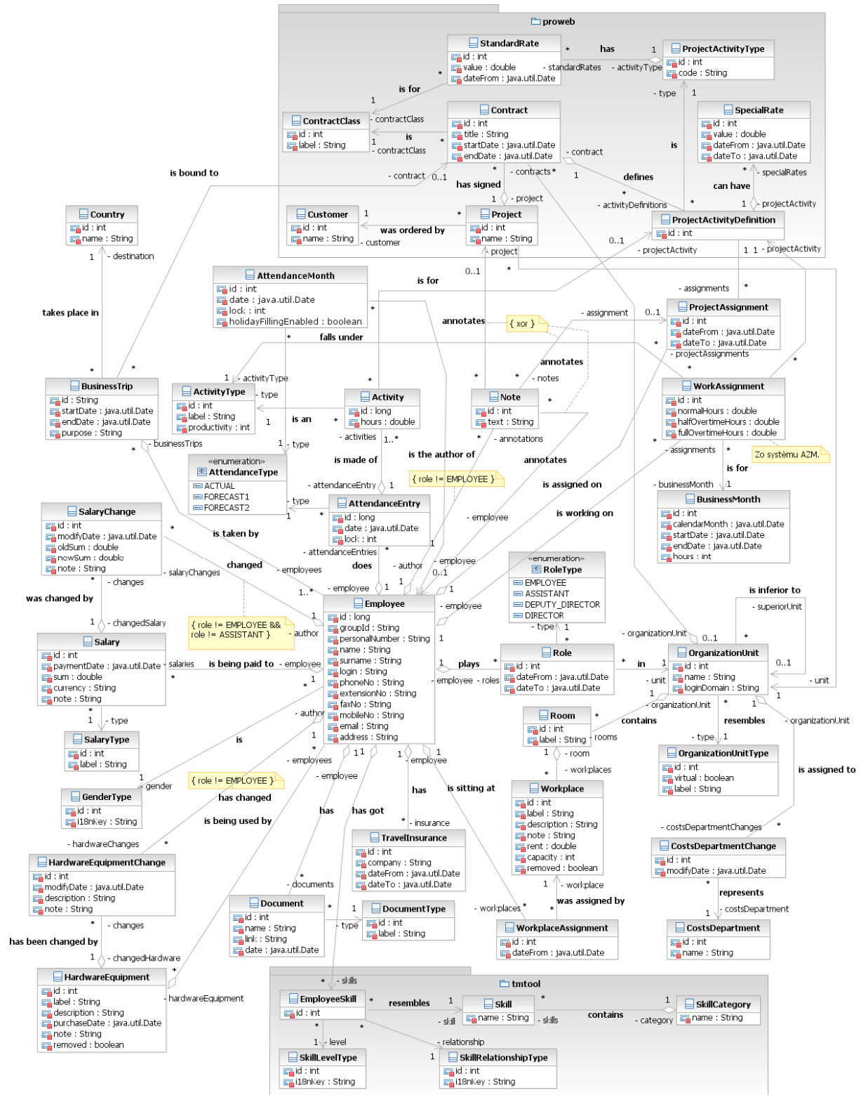
Obr. 68. Reálny fyzický model údajov.
