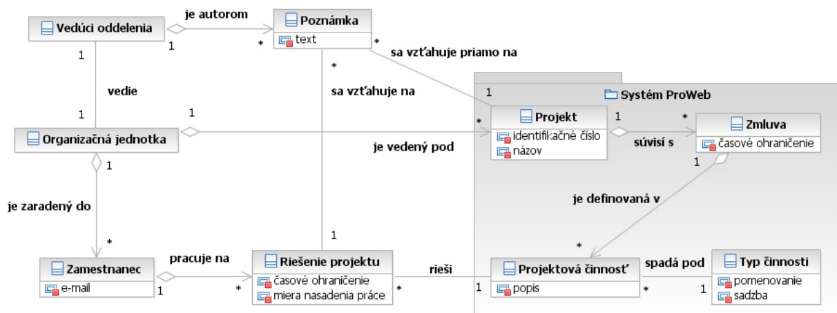
Obr. 41. Logický model údajov pre časť Manažment projektov.
